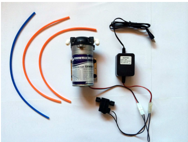
GMWROPUMPKIT – KIT de BOMBA DE PRESION: para instalaciones con poca presión. Válida para POWER GROW y MAXQUARIUM.
