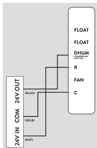
SCHALTPLAN FÜR QUEST CLOUD CONTROL
