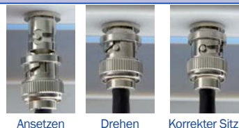
Anschließen des Bluelab pH Probe an das Messgerät
