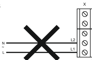
Wiring diagram 15
